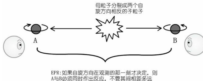
图8.5 EPR佯谬
