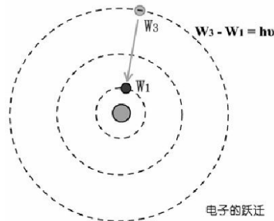
图3.11 玻尔原子中的电子跃迁
