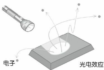
图3.1 光电效应
