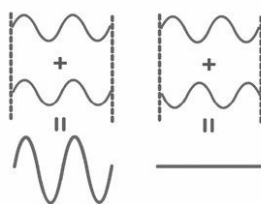
图1.8 波的叠加
