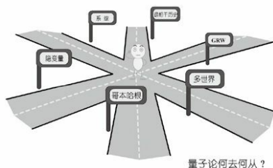
图12.6 量子论迷宫
