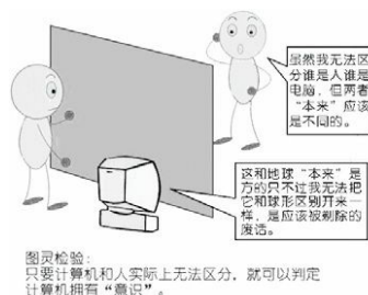
图9.5 图灵检验
