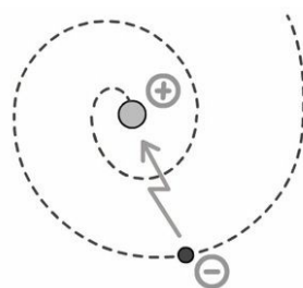
电子和原子核之间释放电磁辐射而导致坠毁
