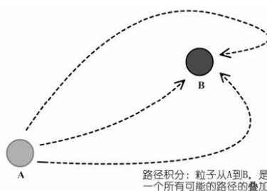
图12.3 路径积分
