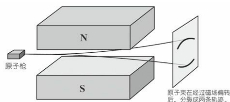
图4.2 斯特恩—盖拉赫实验示意图
