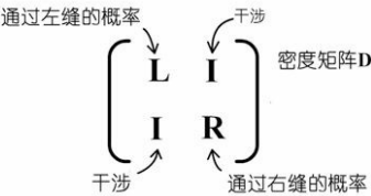
图12.2 密度矩阵
