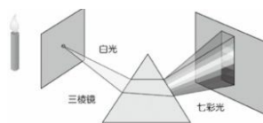
图1.6 光的色散
