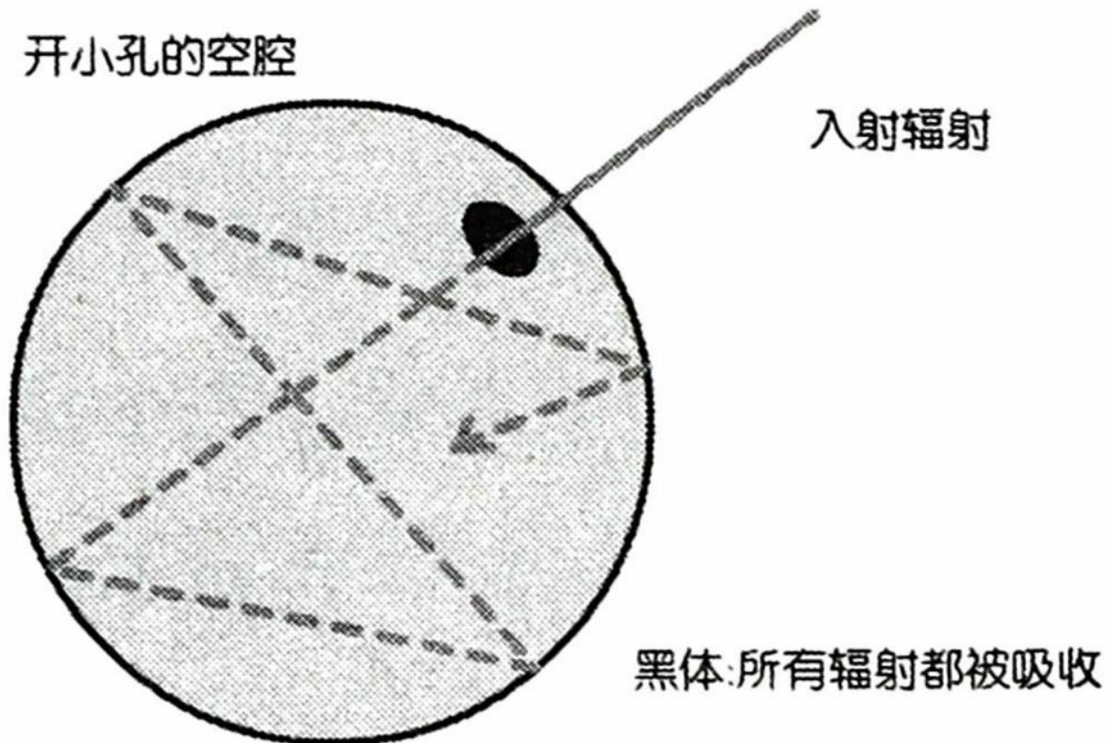
图2.3 黑体
