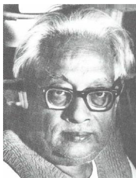
图4.10 玻色
