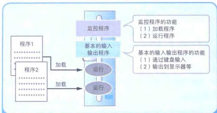
图 9-2 初期的操作系统 = 监控程序 + 基本的输入输出程序
