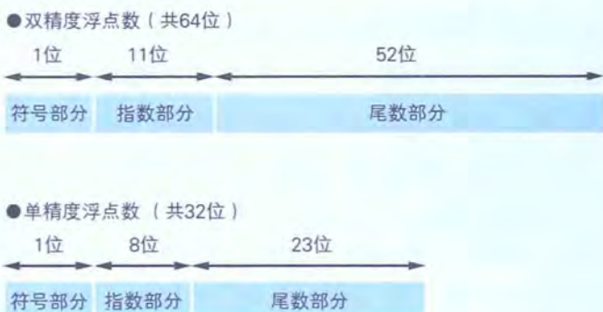
图 3-4 浮点数的内部构造 (IEEE 的规定)
