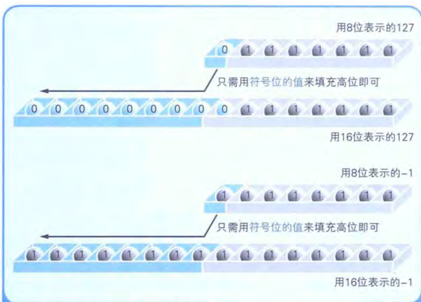
图 2-11 由 8 位转换成 16 位的符号扩充方法
